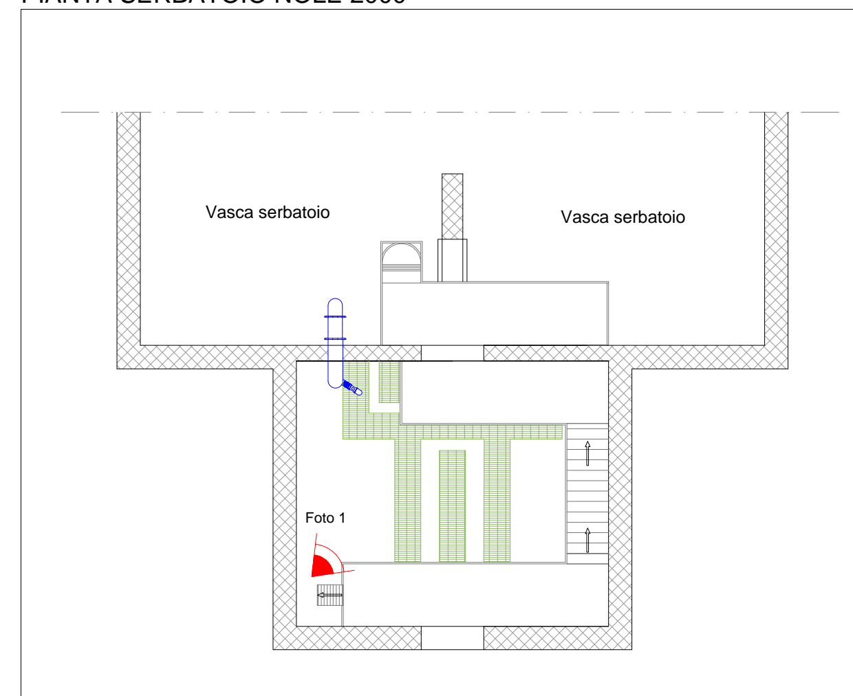
SCHEMA TUBI SERBATOIO NOLE 2000
