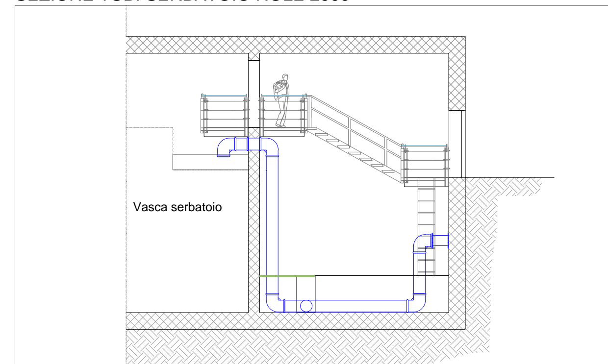
SERBATOIO ESISTENTE NOLE 2000
