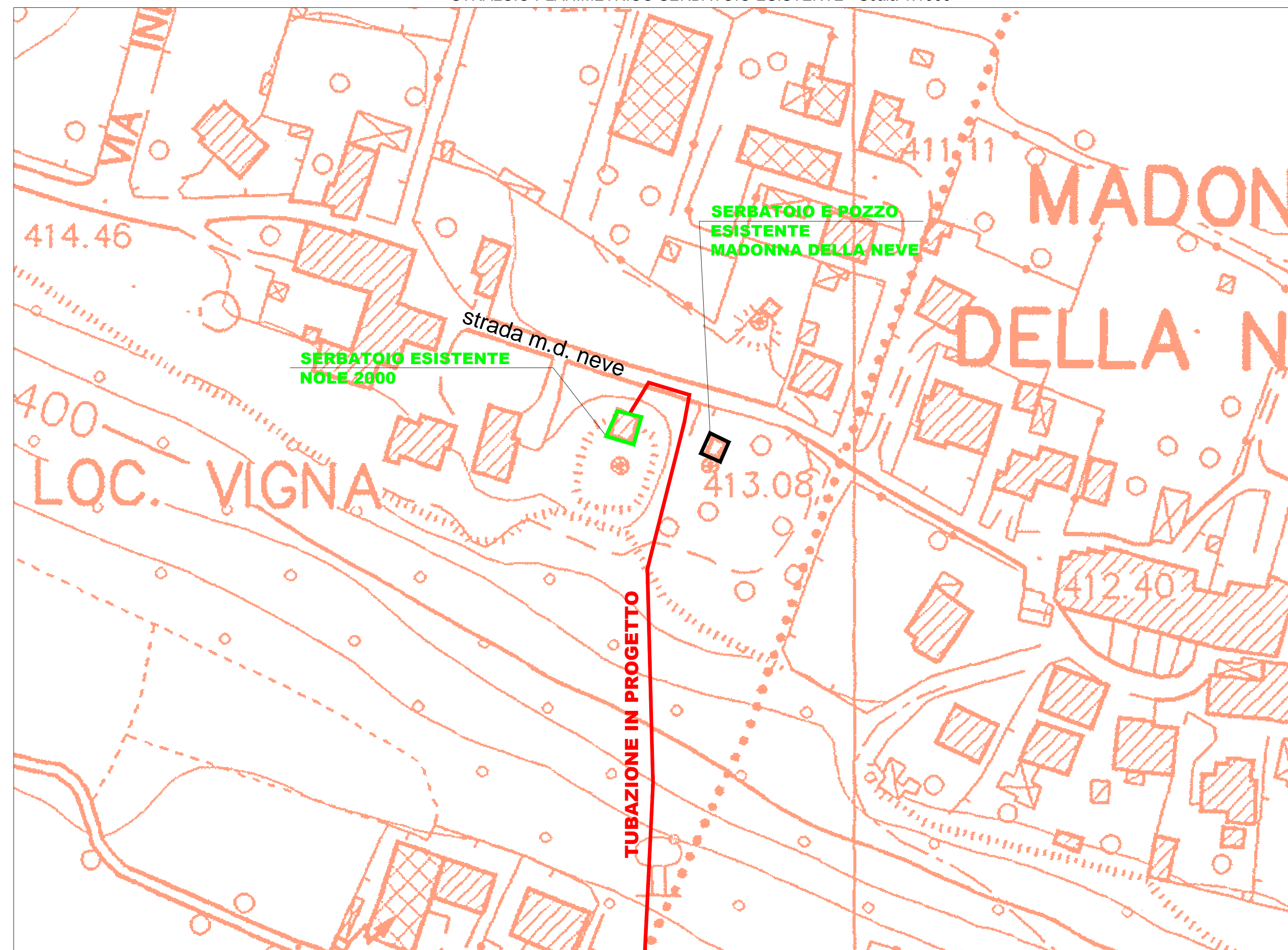
STRALCIO PLANIMETRICO SERBATOIO ESISTENTE - Scala 1:1000
