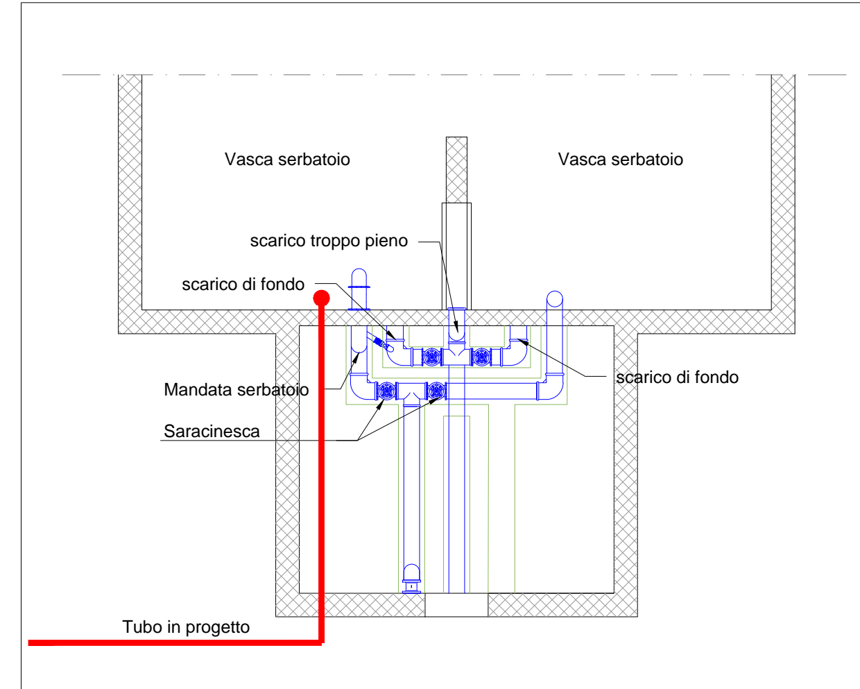
SEZIONE TUBI SERBATOIO NOLE 2000
