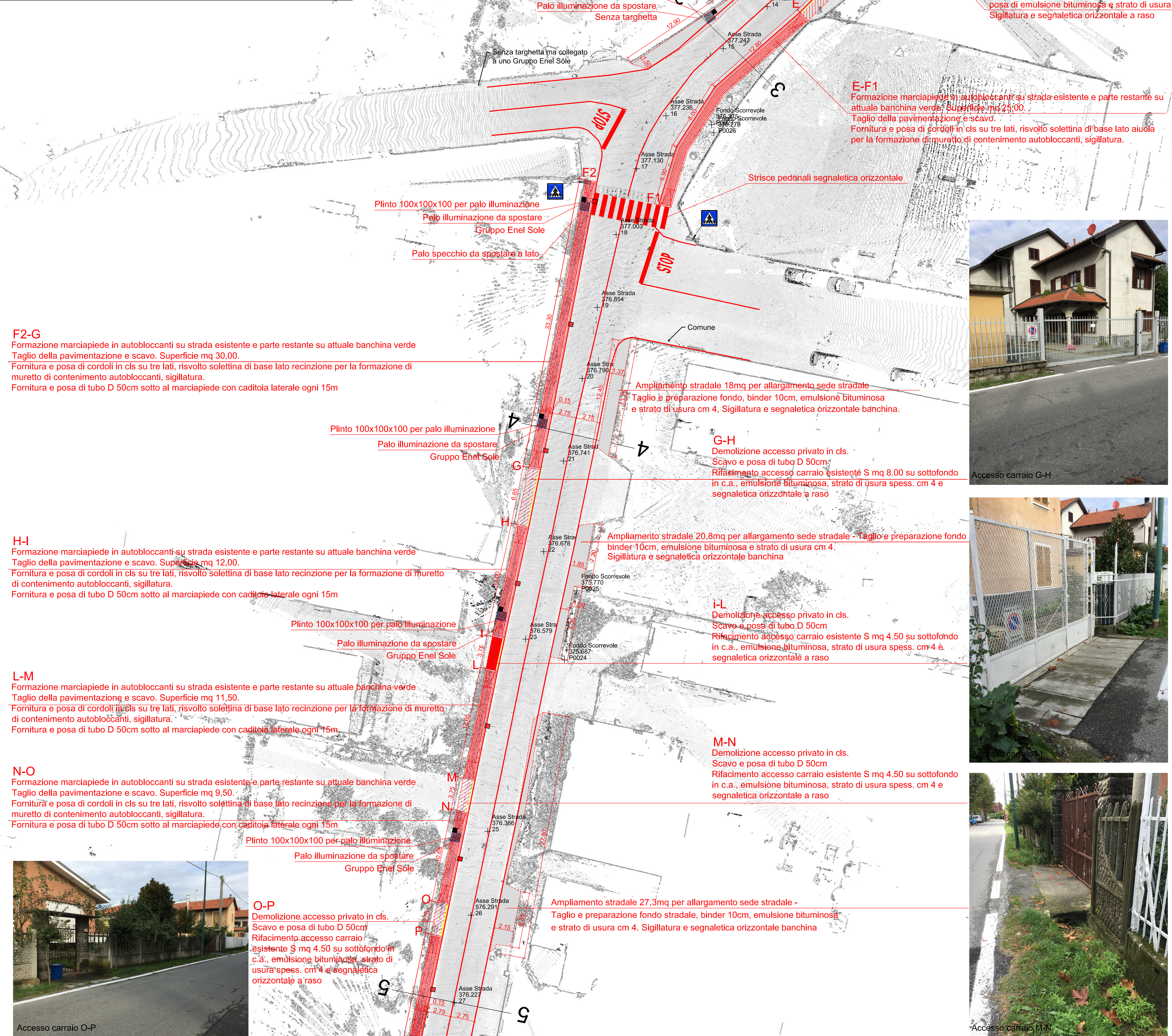
Dettagli costruttivi - scala 1:20
