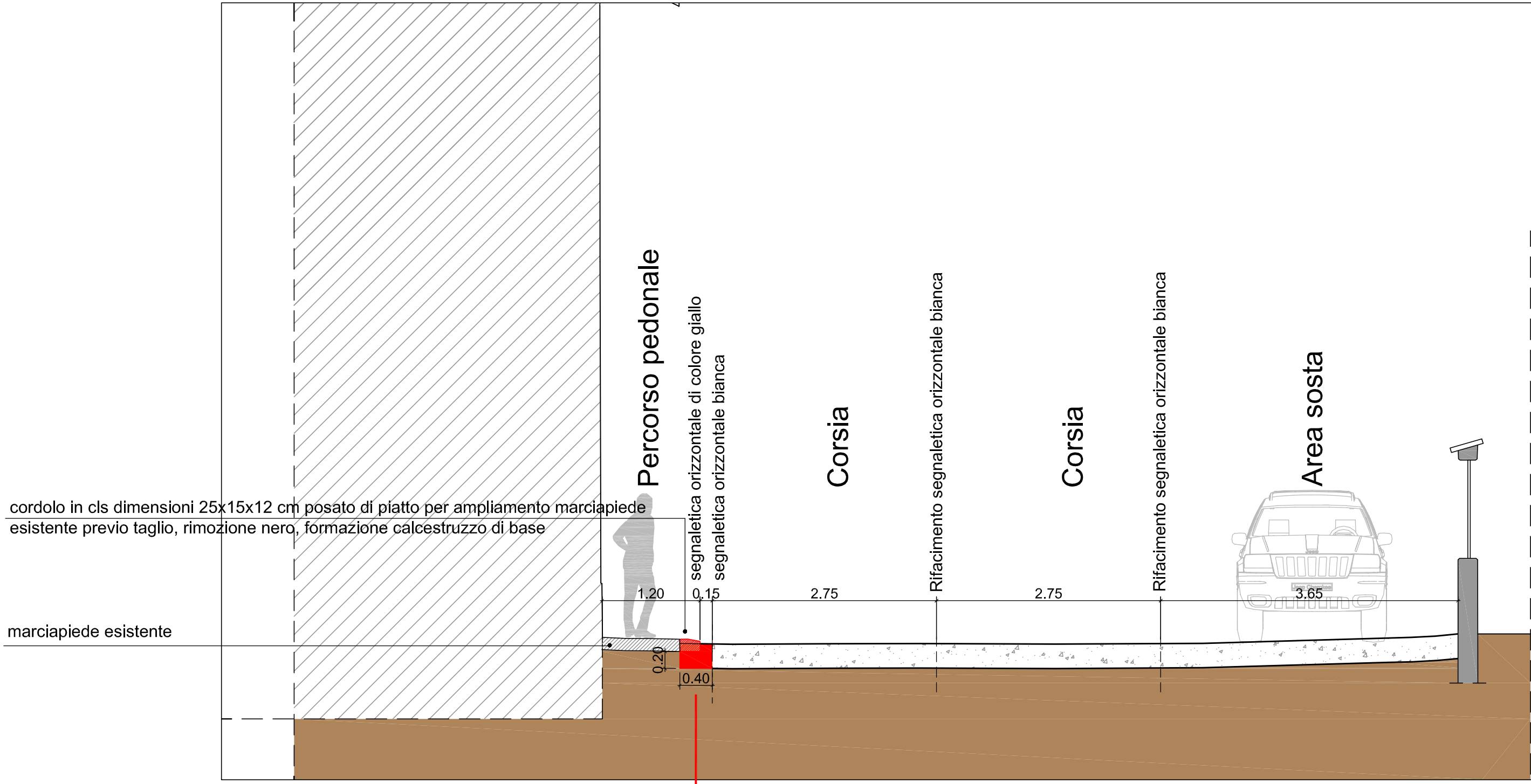
Via I° Maggio - Sezione trasversale tipo 2 - scala 1:50
