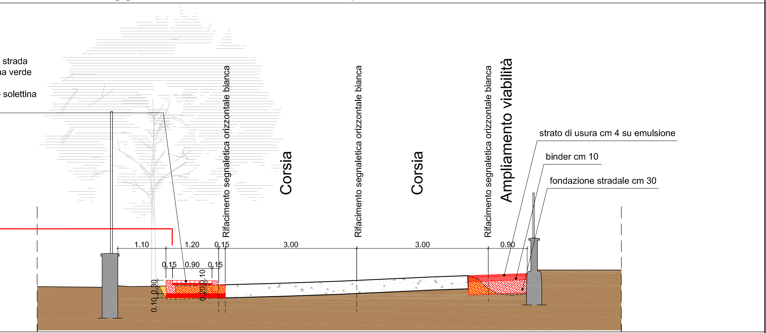
Via I° Maggio - Sezione trasversale tipo 3 - scala 1:50
