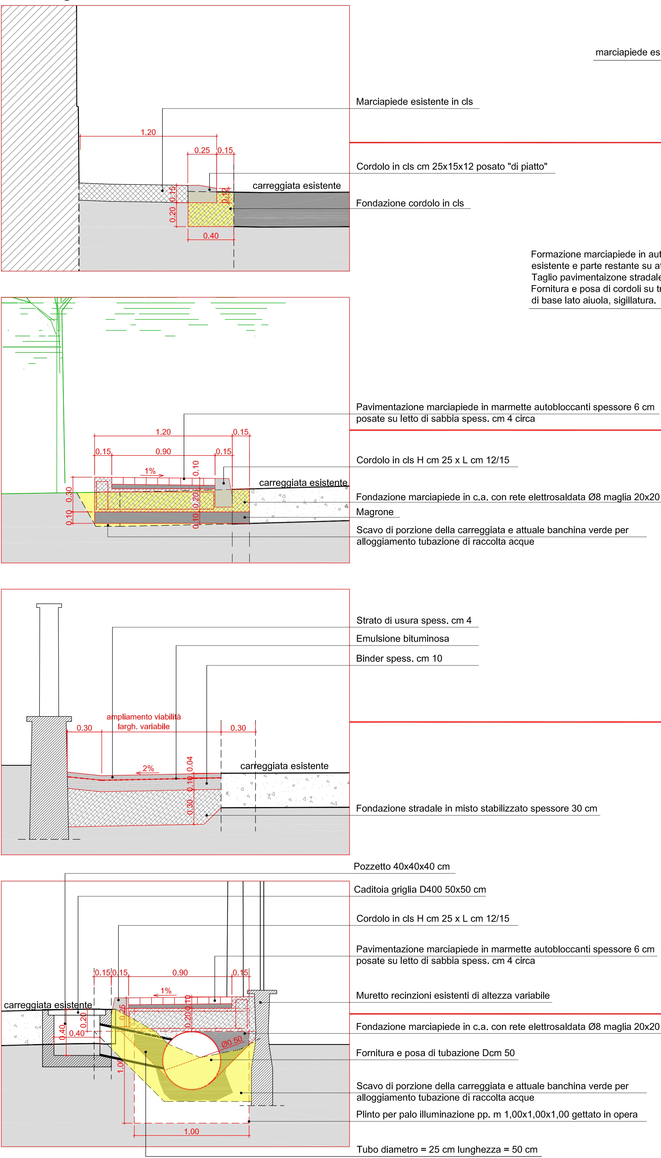
Dettagli costruttivi - scala 1:20
