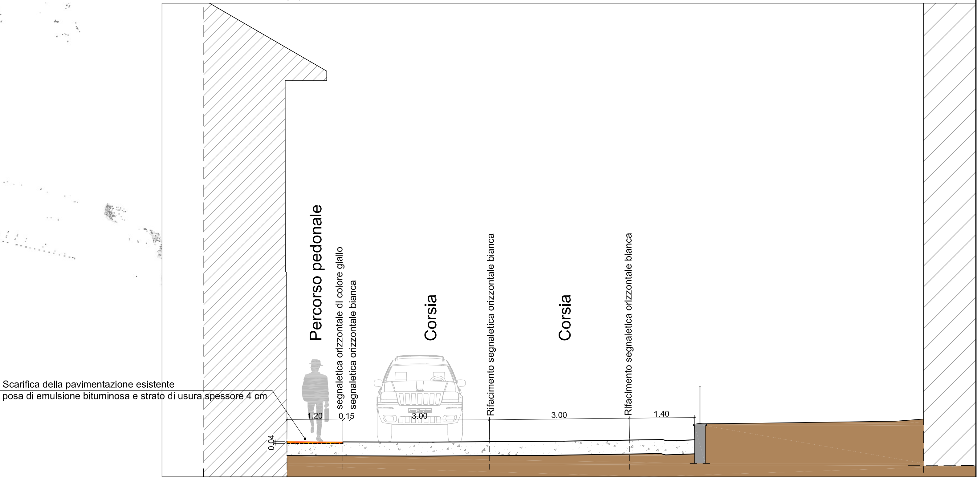
Via I° Maggio - Sezione trasversale tipo 1 - scala 1:50
