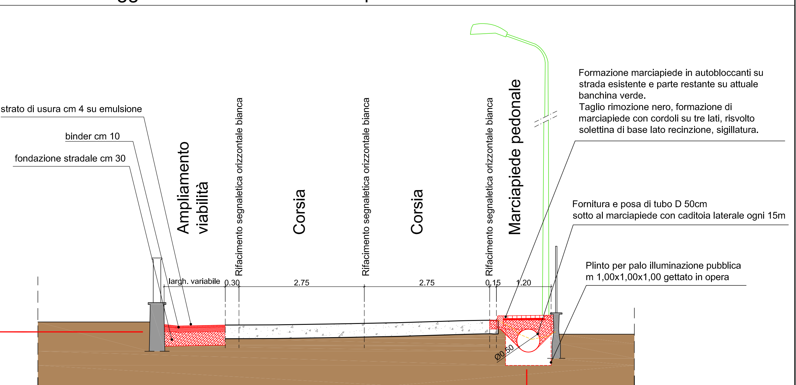
Via I° Maggio - Sezione trasversale tipo 4 - scala 1:50
