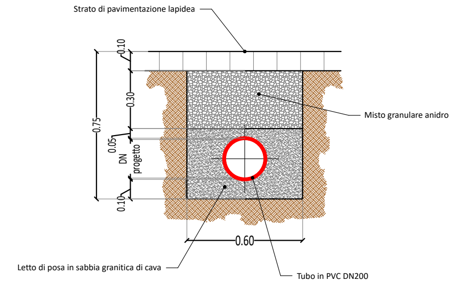
SEZIONE TIPO SU PAVIMENTAZIONE LAPIDEA scala 1:20
