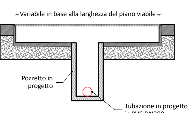
GRIGLIA SEZIONE LONGITUDINALE scala 1:50
