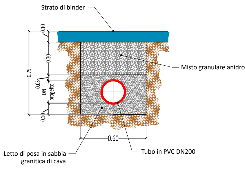
SEZIONE TIPO SU STRADA scala 1:20
