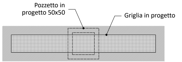
PIANTA GRIGLIA scala 1:50
