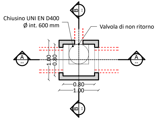
PIANTA GRIGLIA scala 1:50
