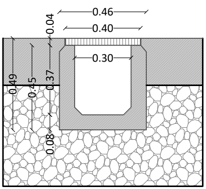
GRIGLIA SEZIONE TRASVERSALE scala 1:20
