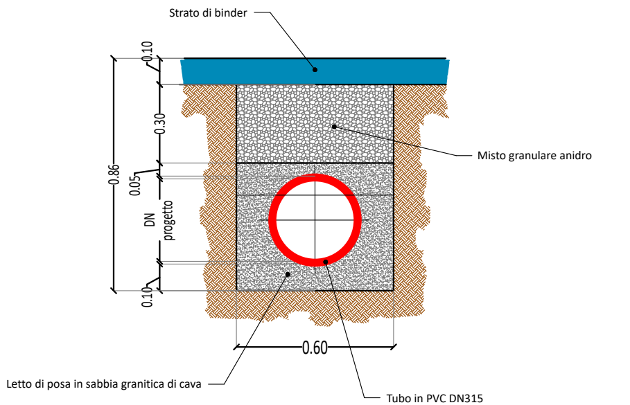
SEZIONE TIPO SU STRADA scala 1:20
