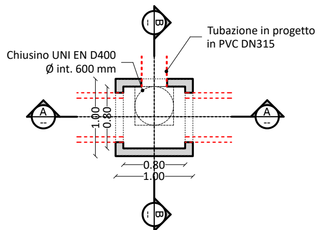
PIANTA ALLACCIO TRATTO 7 scala 1:50
