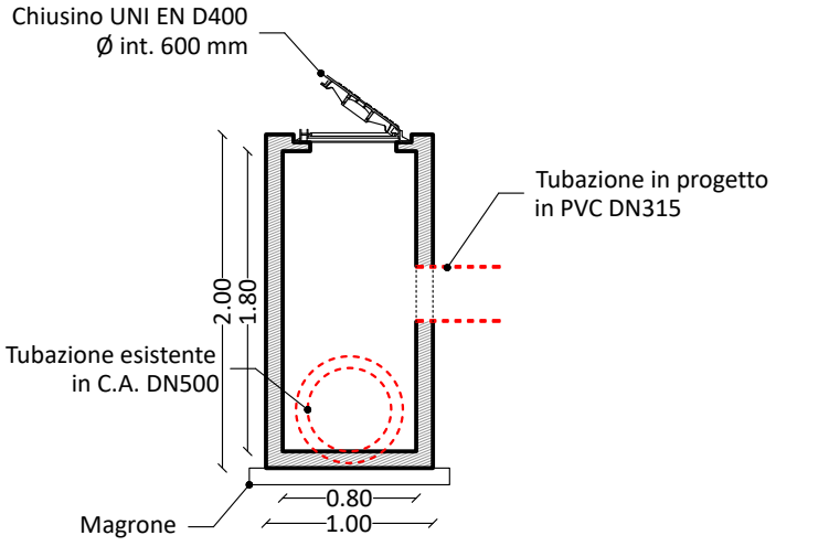
SEZIONE B-B scala 1:50
