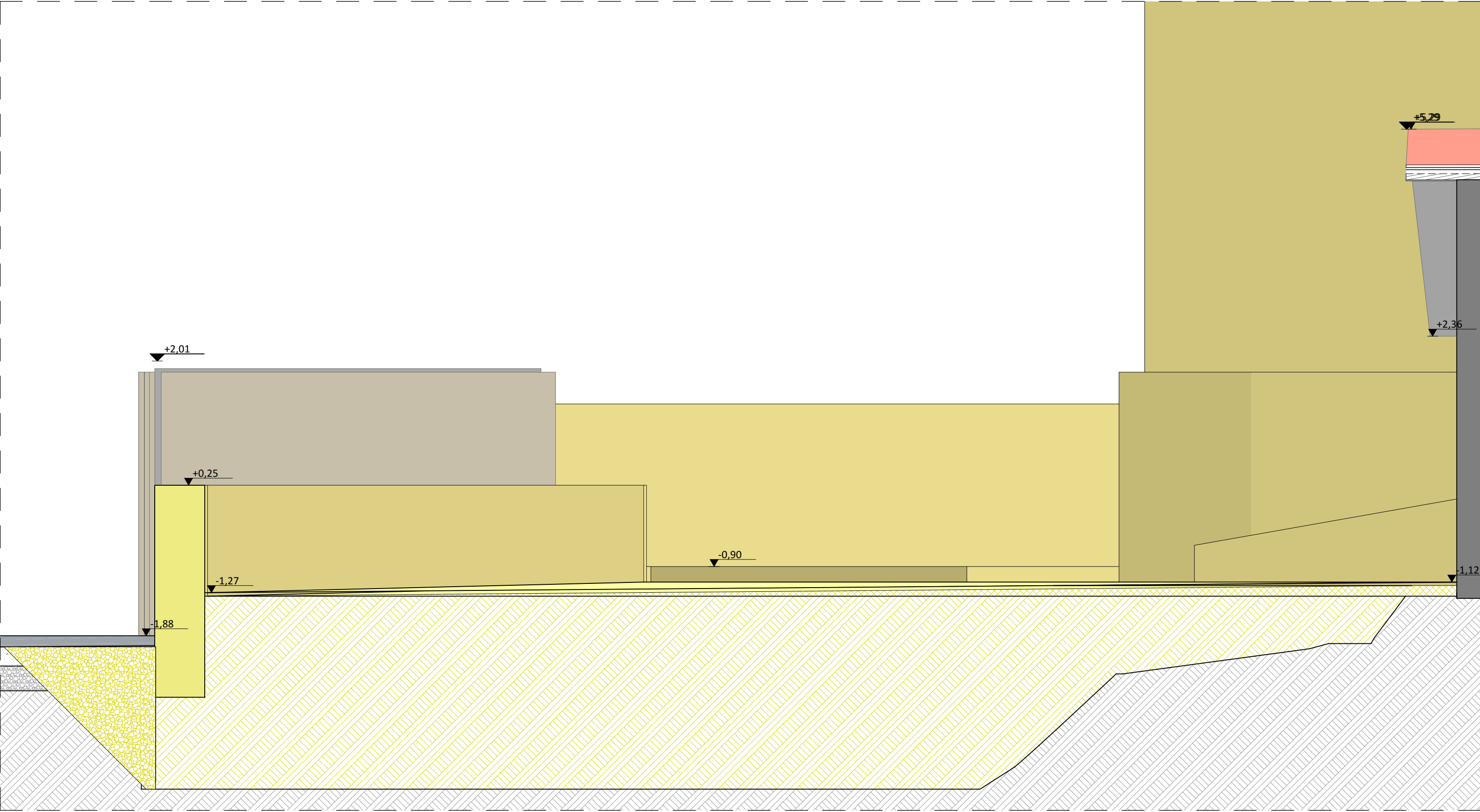
SEZIONE B-B
