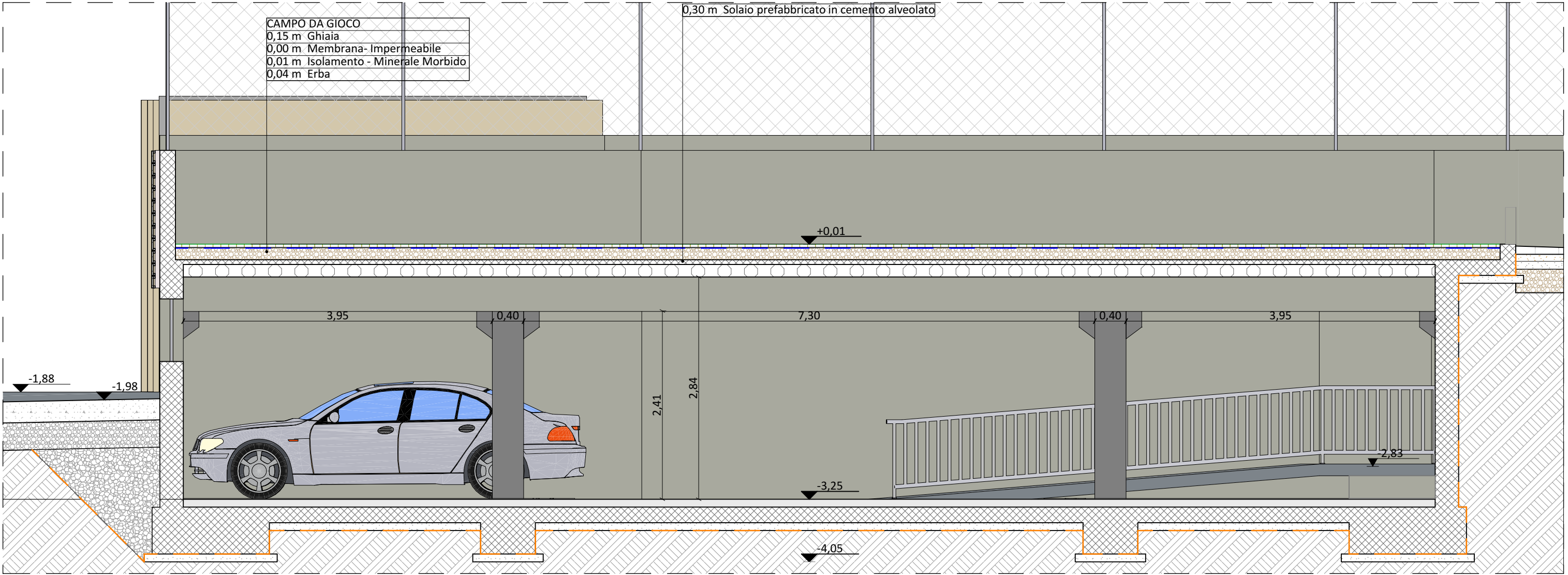
SEZIONE D-D
